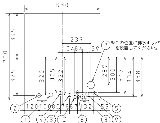
配線・配管立上げ位置図
