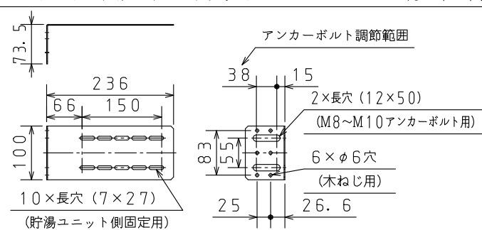
壁固定金具 (別売品) 外形寸法図 (S=1:10)
