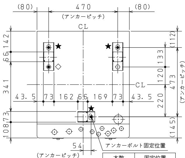
アンカーボルト固定位置図
