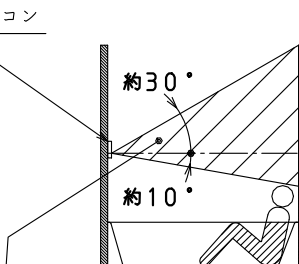
人感センサー検知範囲 (イメージ図)
