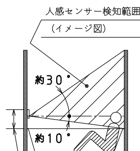
人感センサー検知範囲 (イメージ図) (約350mm以下) リモコン天面～浴槽縁
