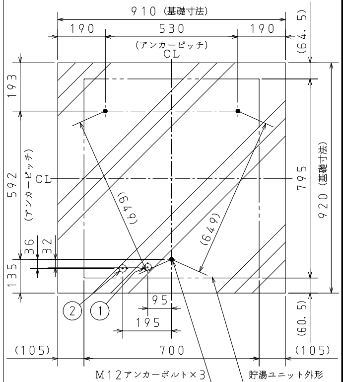
基礎寸法の参考図（地上階設置・独立基礎の場合）
