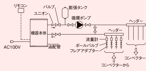
■密閉式温水システムの場合 ※各部材はすべて別売です。
