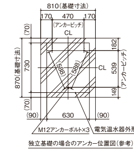
M12アンカーボルト×3 電気温水器外形 独立基礎の場合のアンカー位置図(参考)
