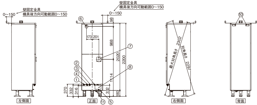
M12アンカーボルト×3 電気温水器外形 独立基礎の場合のアンカー位置図(参考)
