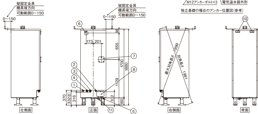
※アンカーボルト固定詳細
