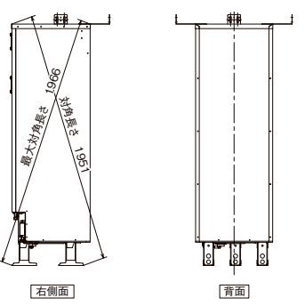
M12アンカーボルト×3 電気温水器外形 独立基礎の場合のアンカー位置図(参考)
