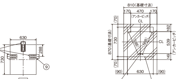
M12アンカーボルト×3 電気温水器外形 独立基礎の場合のアンカー位置図(参考)
