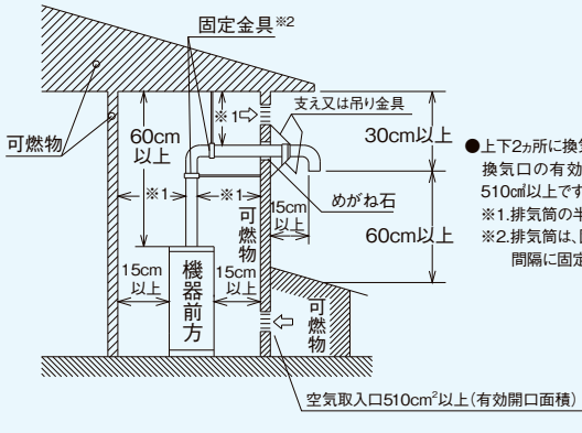
機器側面側に排気筒を設置する場合
