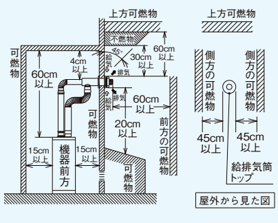
QU8-3LP、QU8-EFLPを使用する場合
