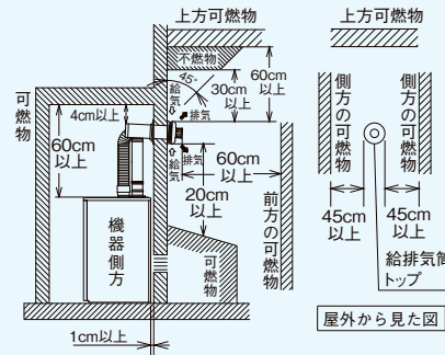
QU8-3SP・QU8-EFSPを使用する場合
