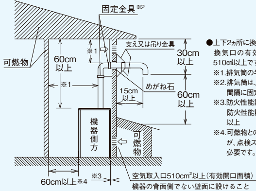
機器背面側に排気筒を設置する場合
