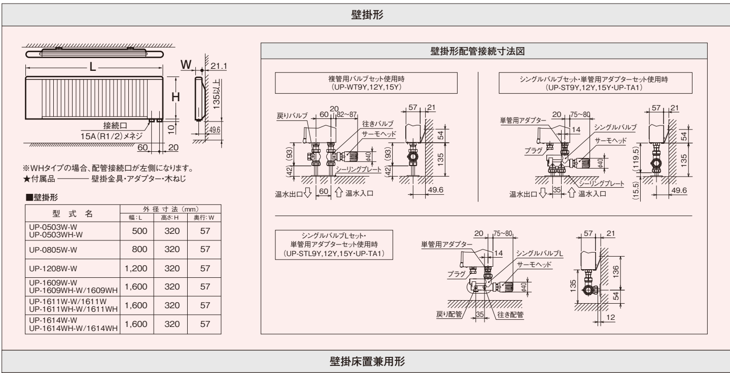
■パネルコンベクターシリーズ寸法図 (単位:mm)
