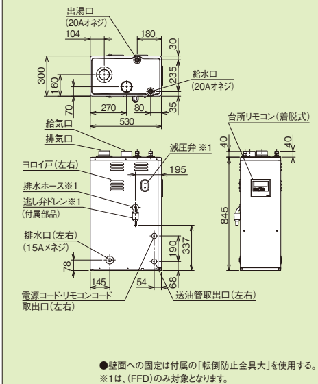
■寸法図(単位:mm)
