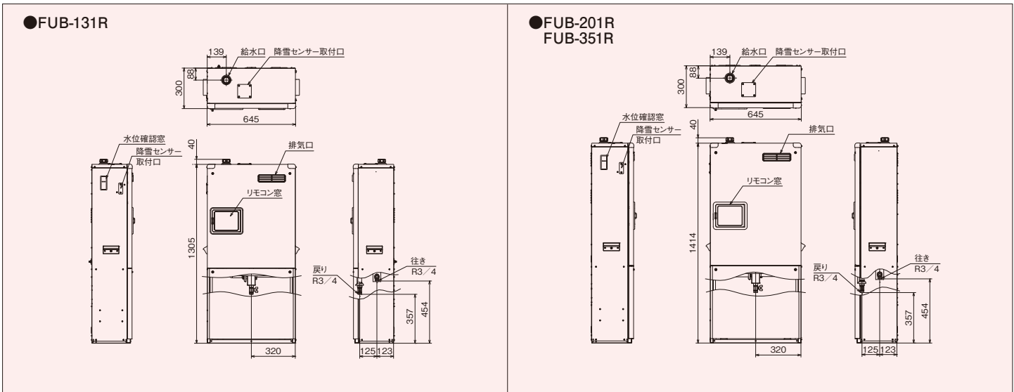
■融雪ボイラー寸法図(単位:mm)
