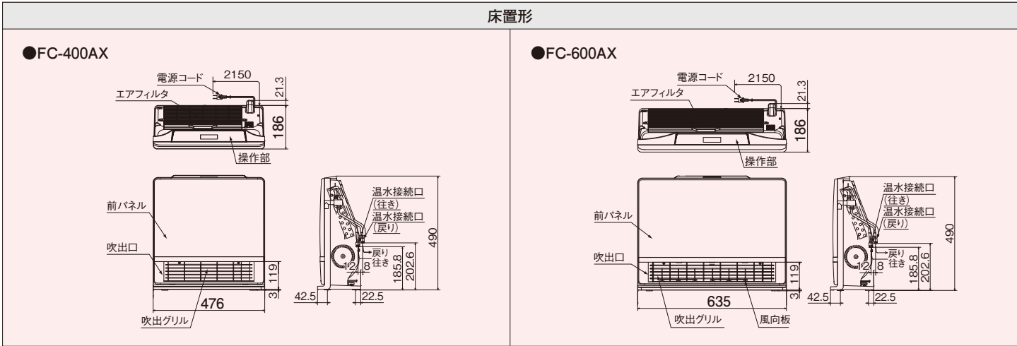
■ファンコンベクター寸法図 (単位:mm)
