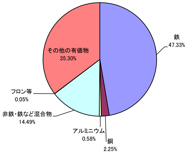
冷蔵庫・冷凍庫の材料構成比
