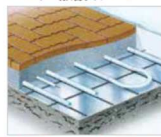
■パイプ敷設イメージ
